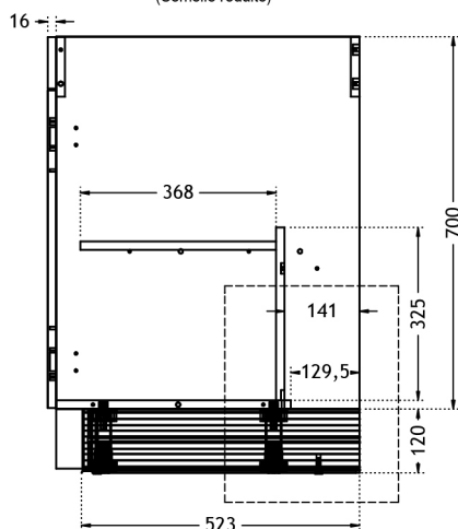
VUE DE DROITE (Semelle réduite)
