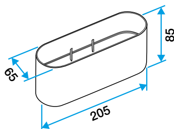
Raccord femelle 60x200 mm
