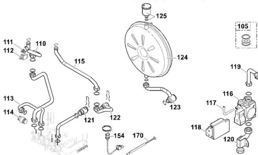
Tubulures / Vanne / Vase d'expansion (City Condens 1.24)
