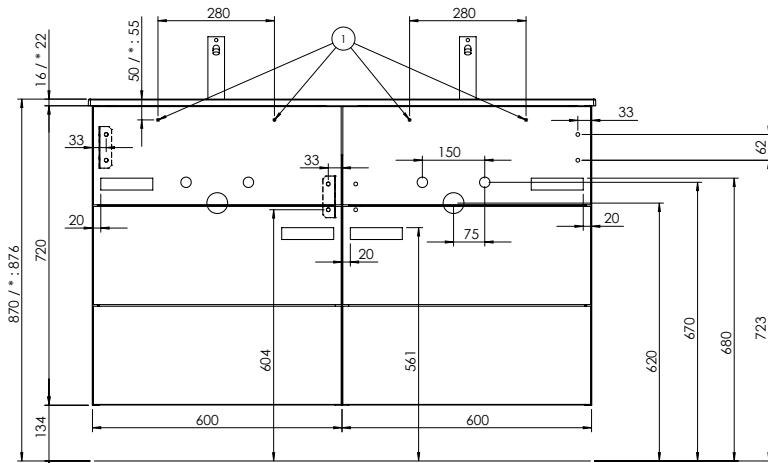
WWYZ120 + MWEB122 / SFPW123 : *
