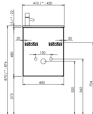
WVWH040 + MWAU042 WVDB040 + SFHH043 : *
