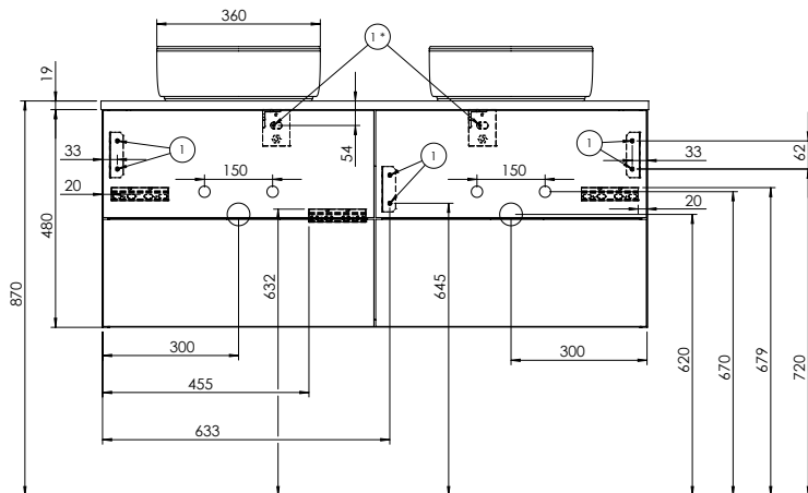
WWDA120 + WPDV120 + SGJQ036 (* : console à placer au plus près de l'axe de la vasque)
