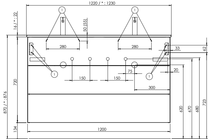
WWYY120 + MWEB122 / SFPW123 : *
