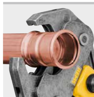
Pince à sertir REMS (4G)
