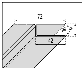
PROFILÉ DE SÉRIE fixation latérale au mur pour tous les modèles
