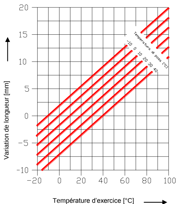
Graphique 3 – Dilatation de 1 m de tube RBM Kilma-Flex PE-RT BAO
