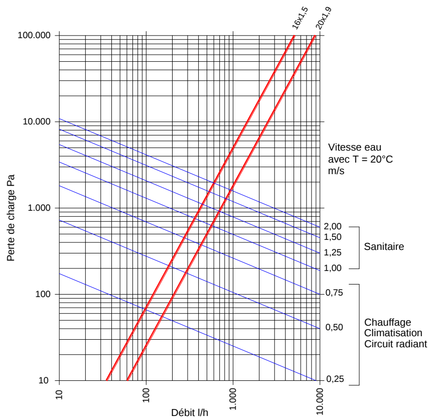
Graphique 4 – Pertes de charge dans le tube RBM Kilma-Flex PE-RT BAO
