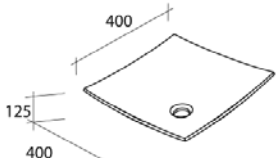
Réf. 121437 Vasque Mini Rialto (sans trop plein) PDS : 8 kg Mini Rialto basin 15 3/4"X 15 3/4" X 5" Waschschale Mini Rialto ohne Überlauf
