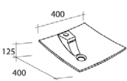
Réf. 121436 Vasque Mini Rialto (avec trop plein) PDS : 8,3 kg Mini Rialto basin (with overflow) 15 3/4"X 15 3/4" X 5" Waschschale Mini Rialto mit Hahnbank und Überlauf
