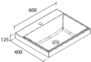
Réf. 1816351 Vasque ALMA Céramyl® Livré sans trop plein et sans kit trop plein 23 5/8" x 15 3/4" x 4 15/16" PDS : 12 kg Delivered without overflow or overflow kit
