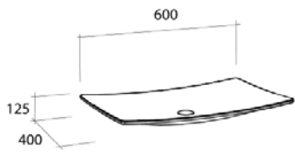
Réf. 121428 Vasque Rialto L 60 (sans trop plein) PDS : 10 kg Basin Rialto W 60 (without overflow) 23 5/8"X 15 3/4"X 4 7/8" Waschschale Rialto B 60 (ohne Überlauf)
