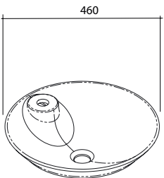
Réf. 1816321 Vasque TULIPE Céramyl® Livré sans trop plein et sans kit trop plein Ø 18 1/8" et H : 4 15/16" PDS : 6 kg Delivered without overflow or overflow kit
