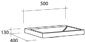
Réf. 1240011 Vasque Séréna semi-encastée (avec trop plein sur l'avant de la vasque) PDS : 10,5 kg Basin Séréna 19 11/16"X 15 3/4" x 5 1/8" Waschschale Séréna mit Überlauf
