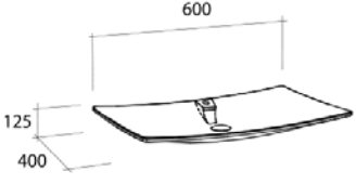
Réf. 121426 Vasque Rialto L 60 (avec trop plein) PDS : 10,3 kg Basin Rialto W60 (with overflow) 23 5/8"X 15 3/4"X 4 7/8" Waschschale Rialto B 60 und Hahnbank(mit Überlauf)
