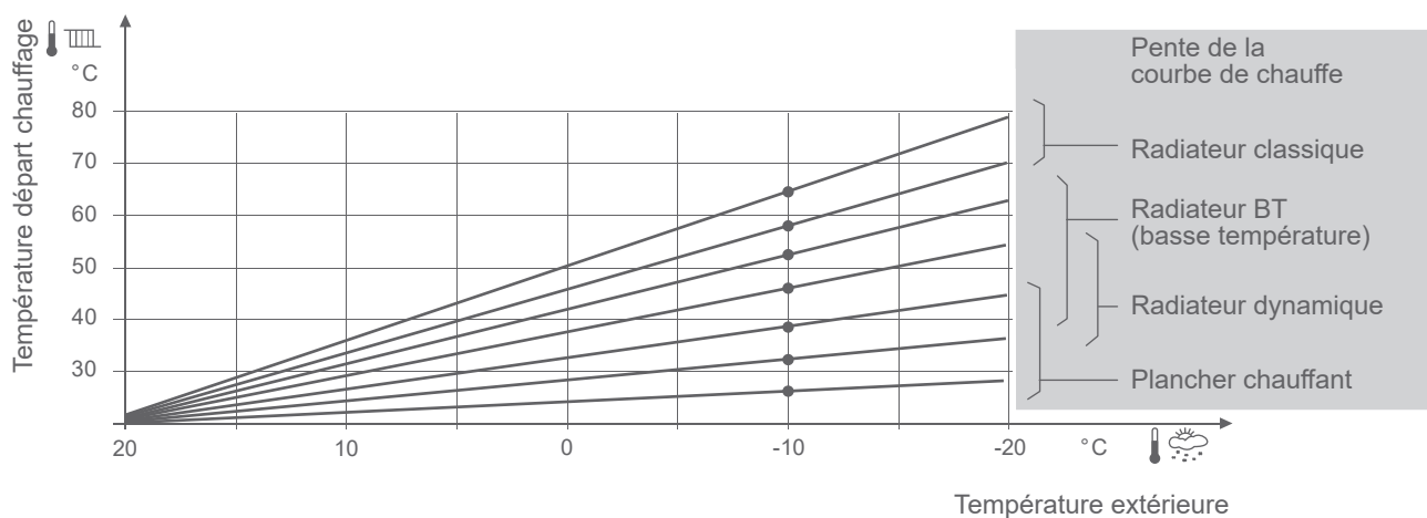
fig. 43 - Pente de la courbe de chauffe
