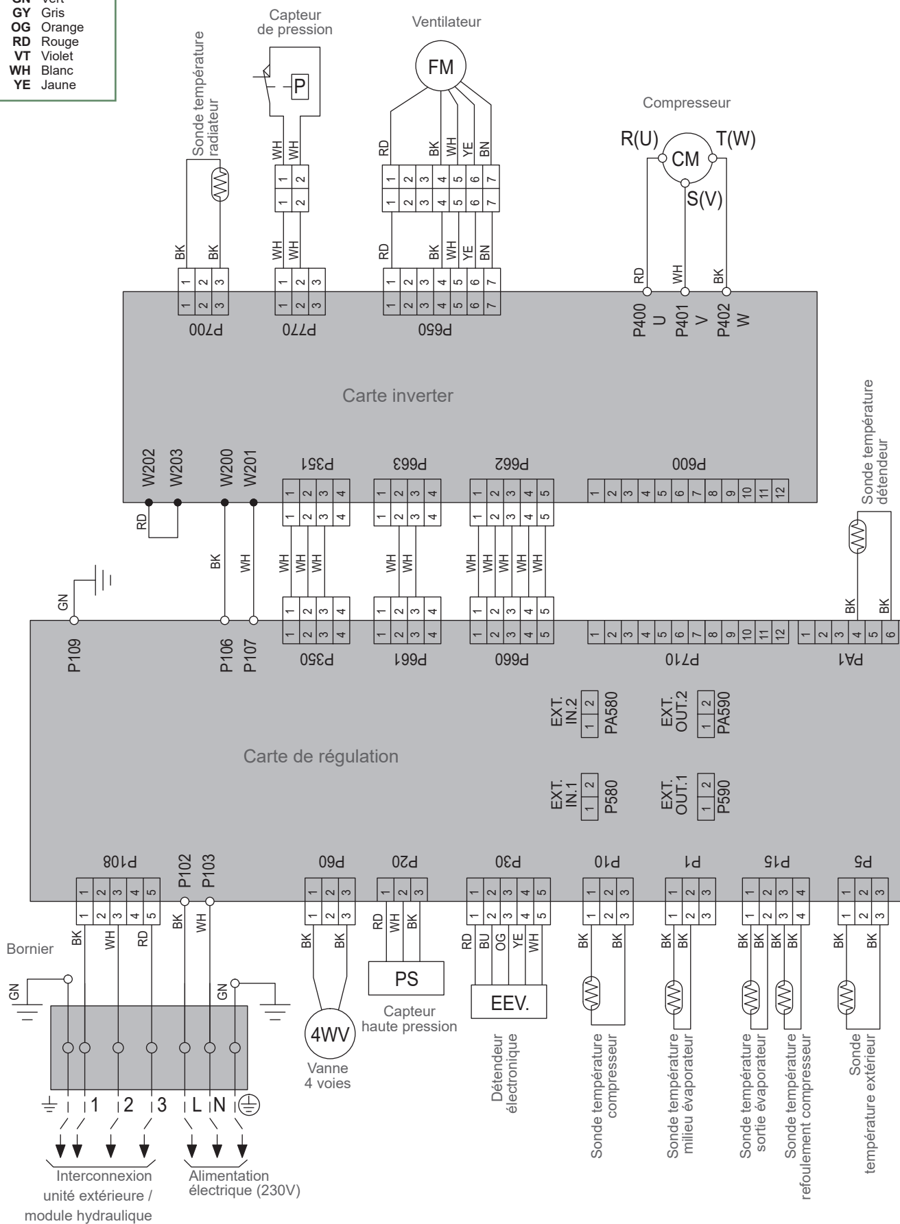
fig. 46 - Câblage électrique unité extérieure modèle 10
