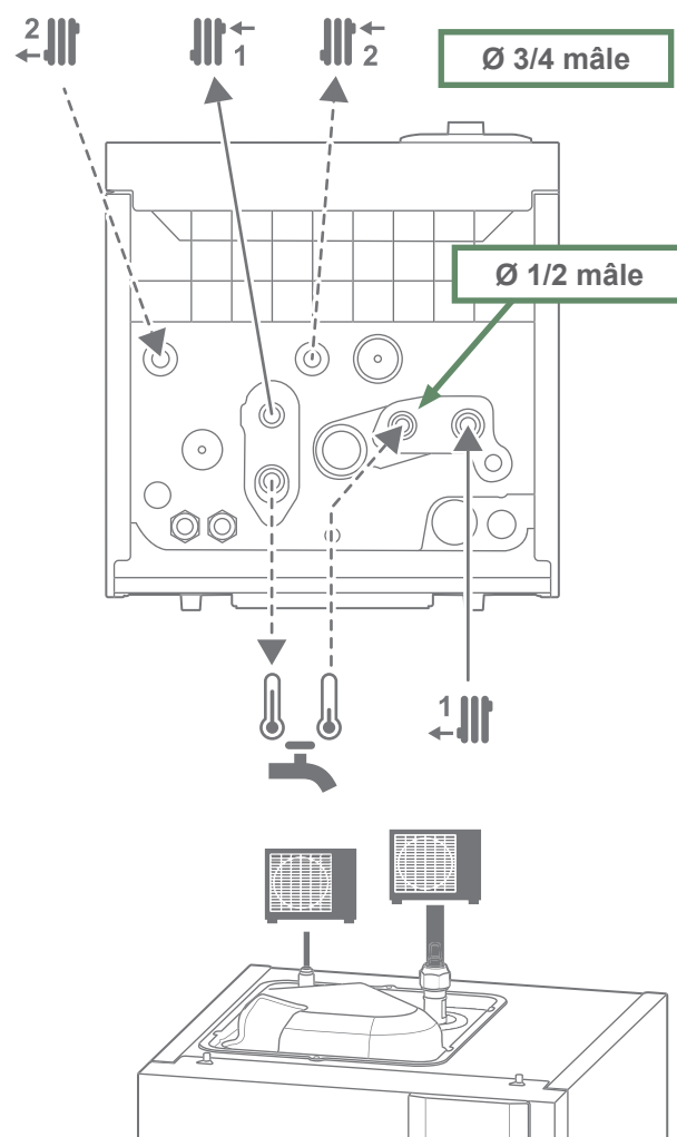
fig. 2 - Repérage hydraulique
