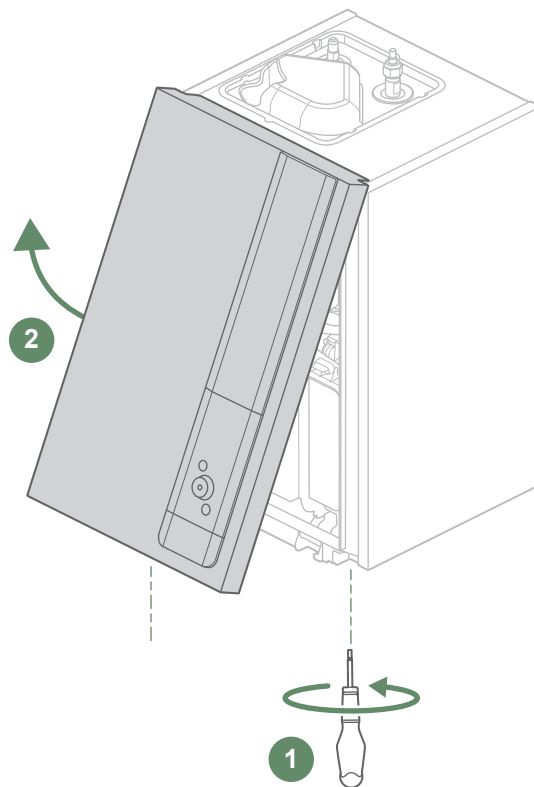
fig. 21 - Ouverture de la façade
