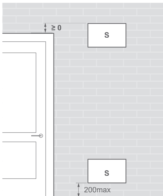
fig. 24 - Position des ouvertures pour la ventilation
