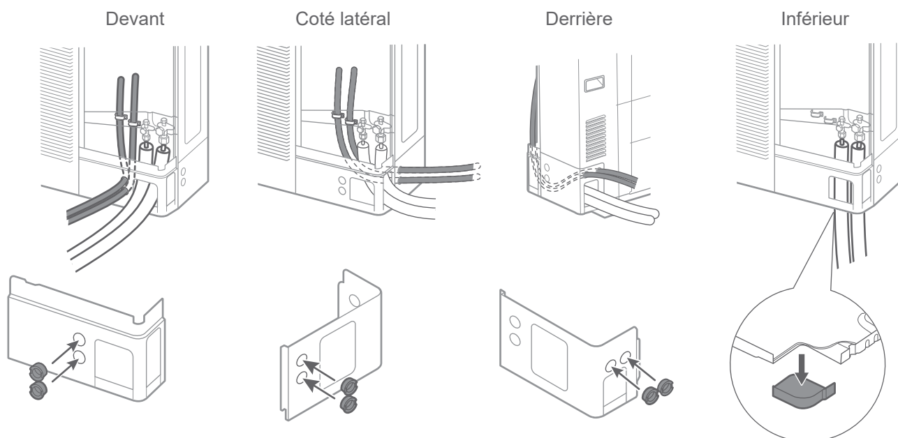
fig. 32 - Passage des liaisons frigorifiques de l'unité extérieure.
