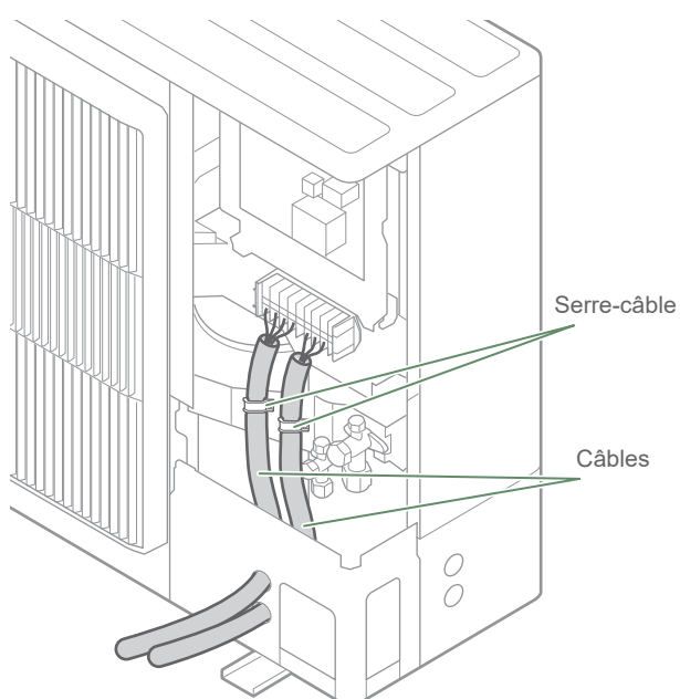
fig. 40 - Accès au bornier de l'unité extérieure
