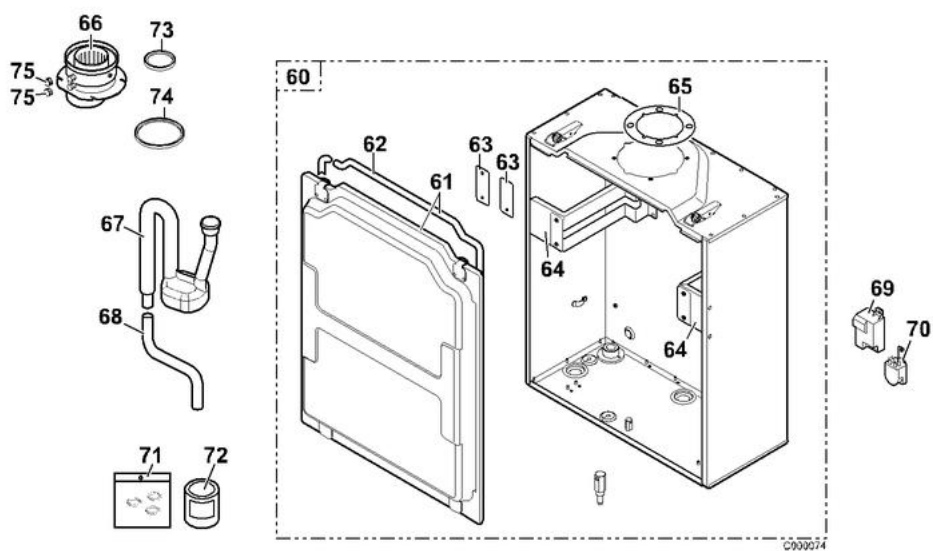
Caisson étanche
