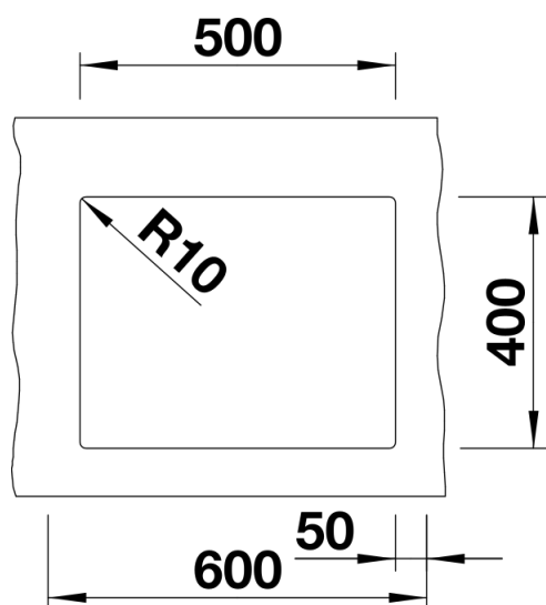
Découpe
