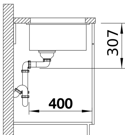
Vue latérale
