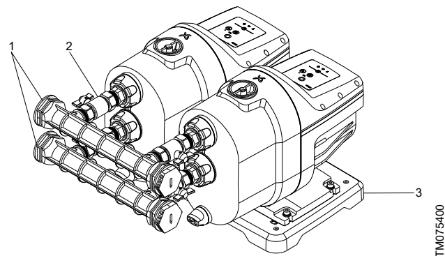
Groupe de surpression double SCALA1
