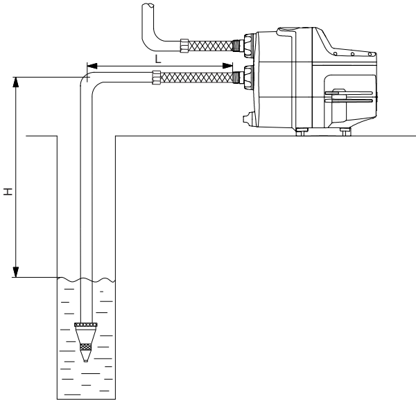
Longueur de la tuyauterie d'aspiration
