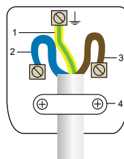
Exemple, câblage d'une fiche
