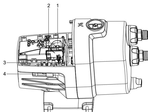
Connexion d'une entrée externe
