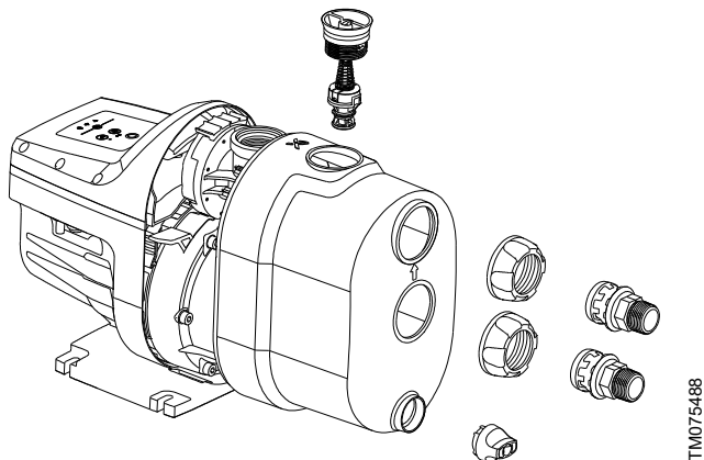
Retrait du couvercle du surpresseur
