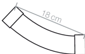
Encombrement coude allongé 45°
