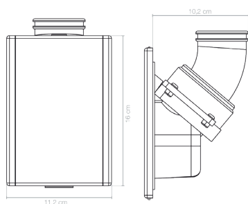
Encombrement prise pour flexible rétractable
