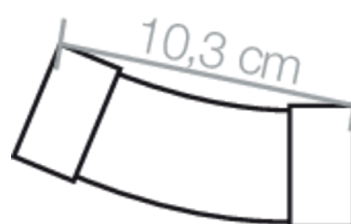
Encombrement coude allongé 22,5°
