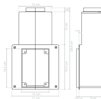
Encombrement contre-prise mur brique pour flexible rétractable
