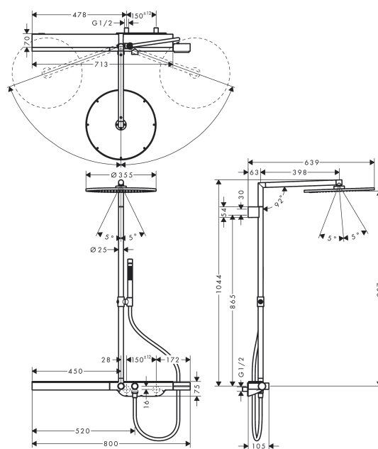
Plan géométral
