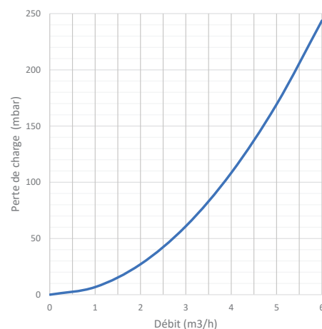
Pertes de charge à débit maximal : 220 mbar
