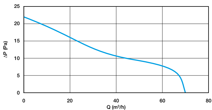
Courbe aérodynamique DECO 100
