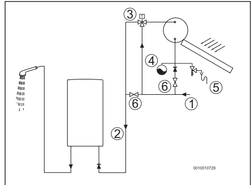
Fig. 18 Installation solaire
