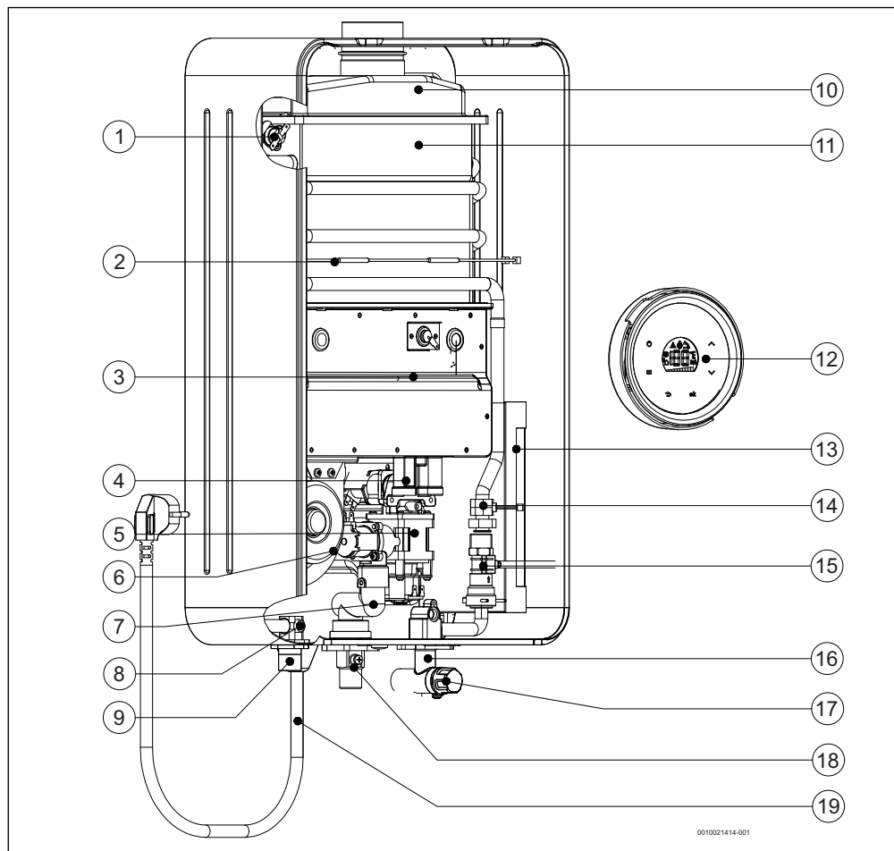
Fig. 2 Aperçu de l'appareil
