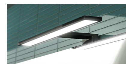
Miroir avec chants finition chromé et attaches réglables. Applique LED basse consommation, disponible en chromé et noir mat (30 W ou 50 W - 4000 K - classe énergétique A).
