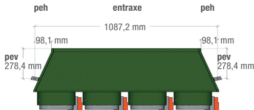
Exemple du schéma du plénum S4 (angle sortant) :
