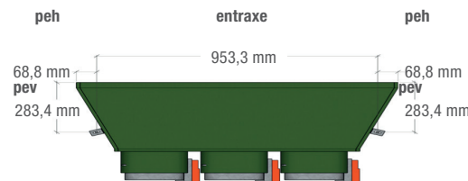
Exemple du schéma du plénum M3 (angle sortant) :
