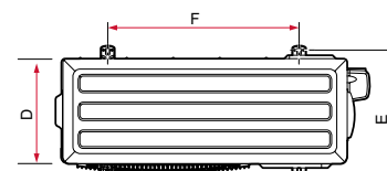
Unité extérieure SDH20-...MC2NO
