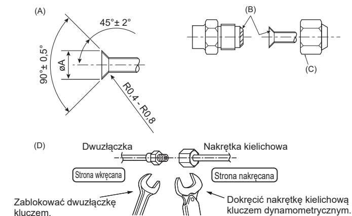
(A) Wymiary przycinania kielichów
