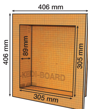
KB 12 N 305 305 A
