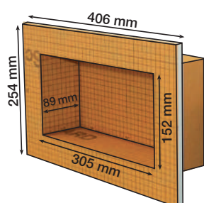
KB 12 N 305 152 A
