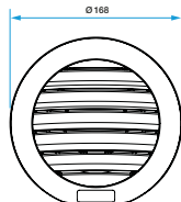
Encombrement Auvent EHT 2 -EFT 2
