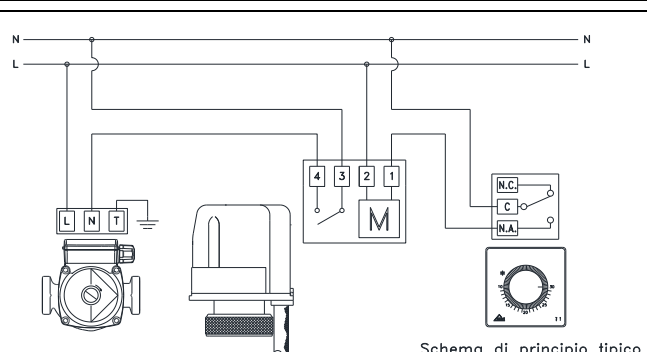
Fig.2 : Câblage électrique de servocommande électro-thermique, avec microrupteur auxiliaire.
