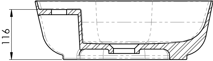
COUPE A-A
