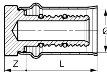
Vue en coupe avec cote
