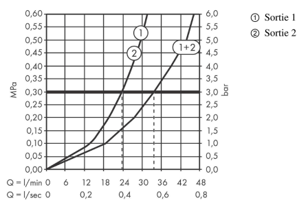
Schéma d'écoulement
