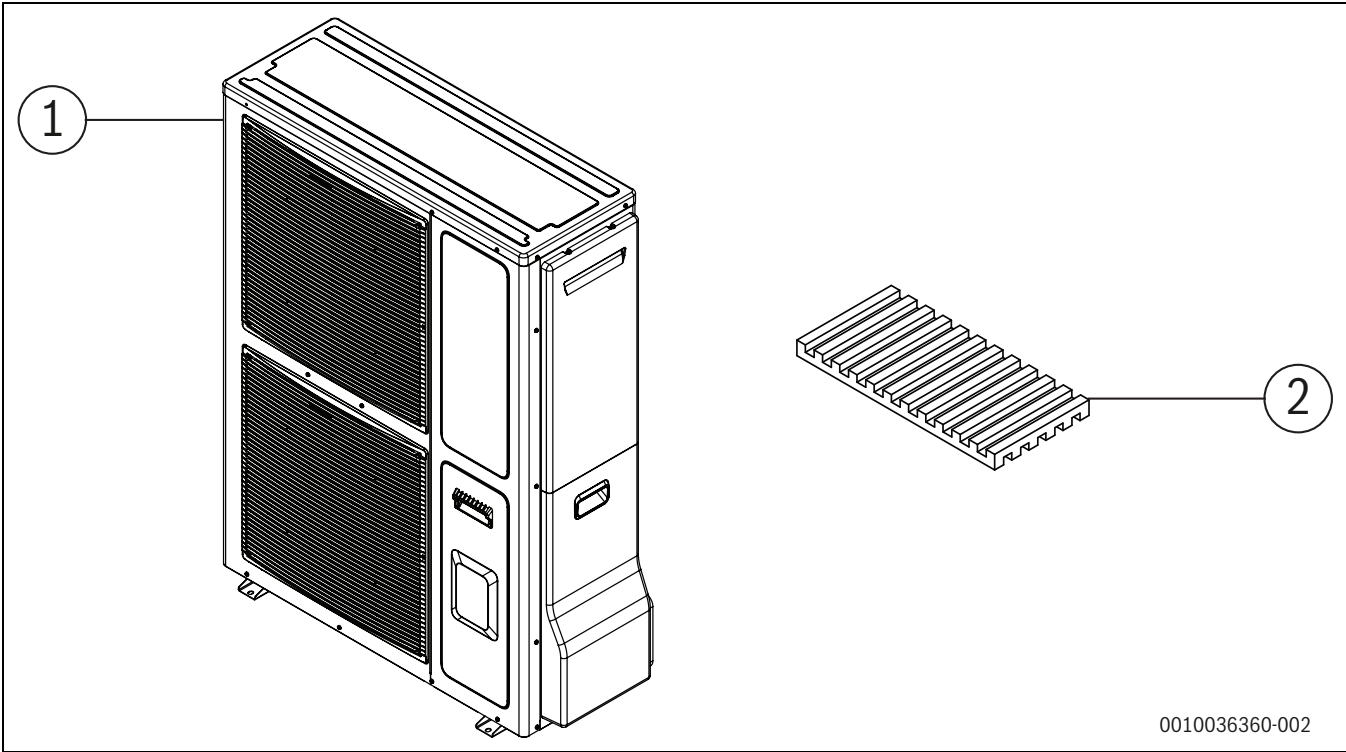
Fig. 1 Pièces fournies
