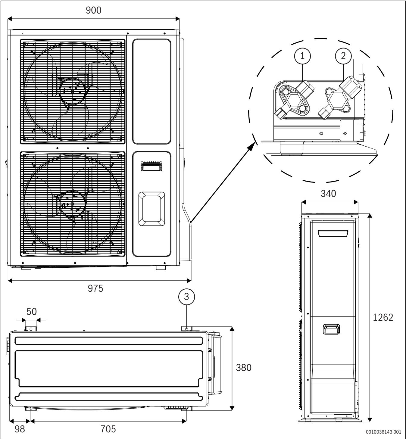
Fig. 2 Dimensions de l'unité extérieure modèle CS3400iAWS 12-14 OR-S et CS3400iAWS 10-14 OR-T
