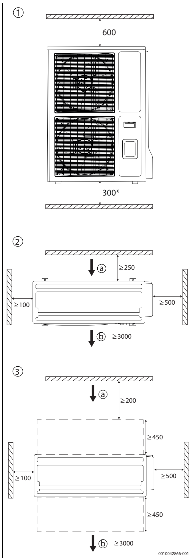
Fig. 3 Dégagements minimaux (mm)
