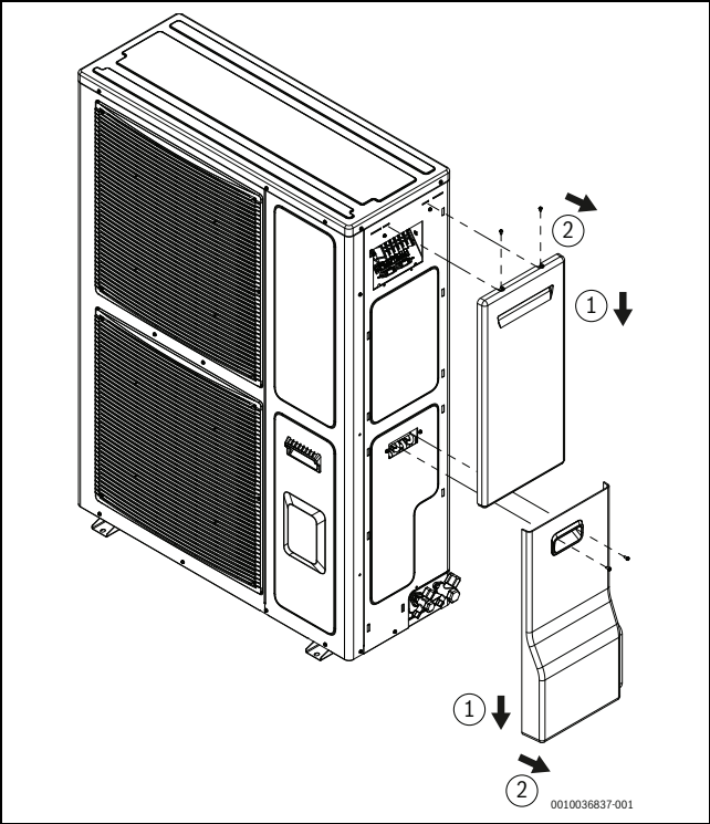
Fig. 12 Retirer le cache latéral
