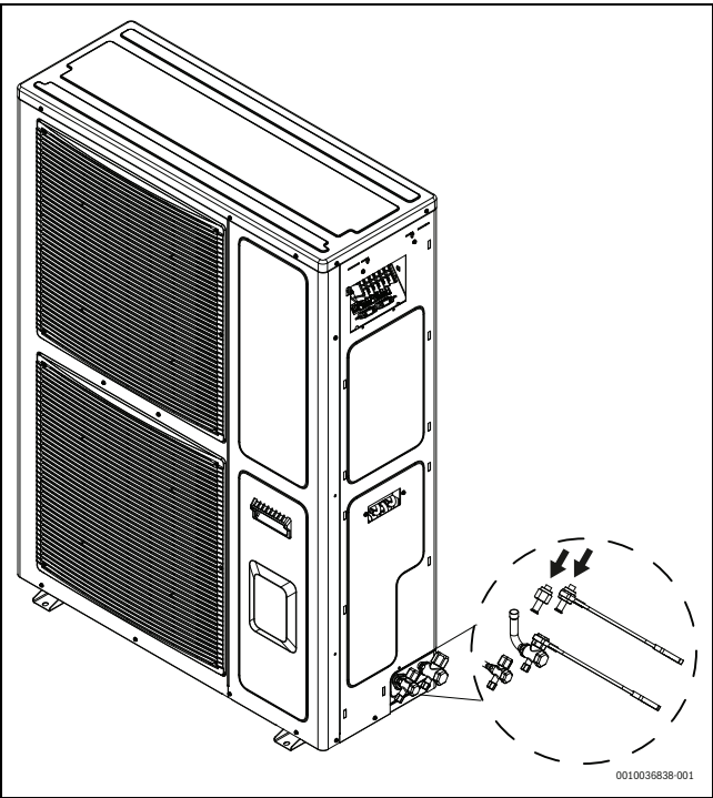
Fig. 13 Vissage
