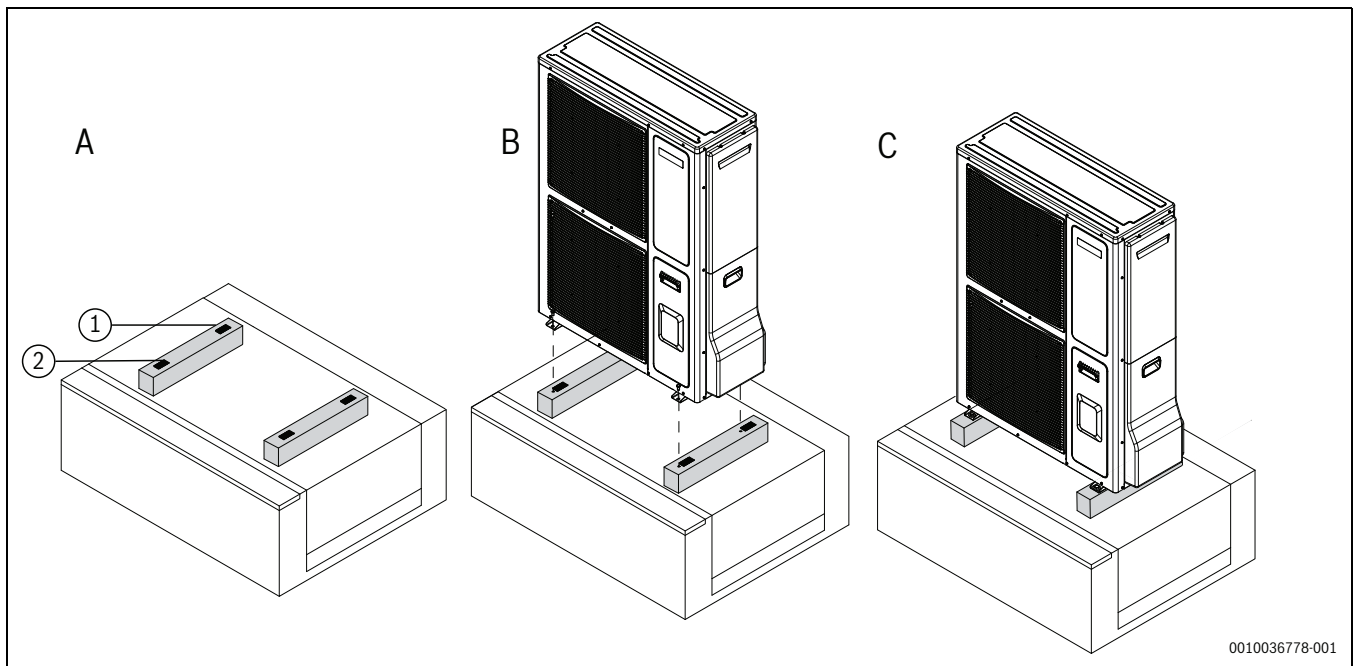
Fig. 7 Unité extérieure au sol
