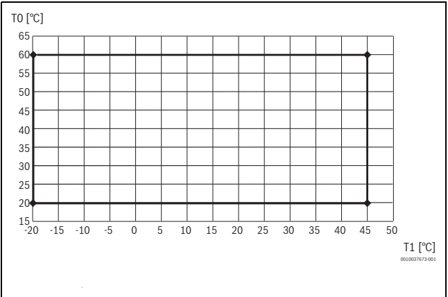
Fig. 23 Plage de fonctionnement de l'unité extérieure en mode chauffage sans chauffage d'appoint pour CS3400iAWS 10-14 OR-T
