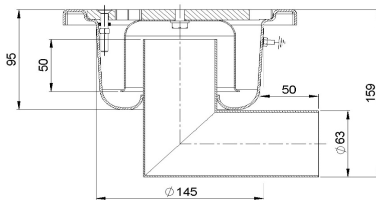
COUPE A-A
