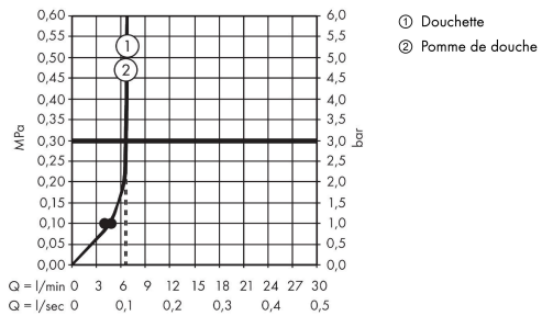
Schéma d'écoulement
