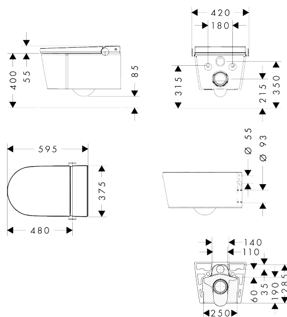
Plan géométral
