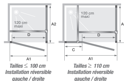
Smart Design P sans seuil (taille ≥ 110 cm) + F sans seuil - profilé chromé
