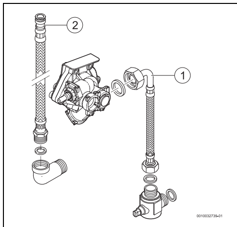
Fig. 12 Raccordement d'eau
