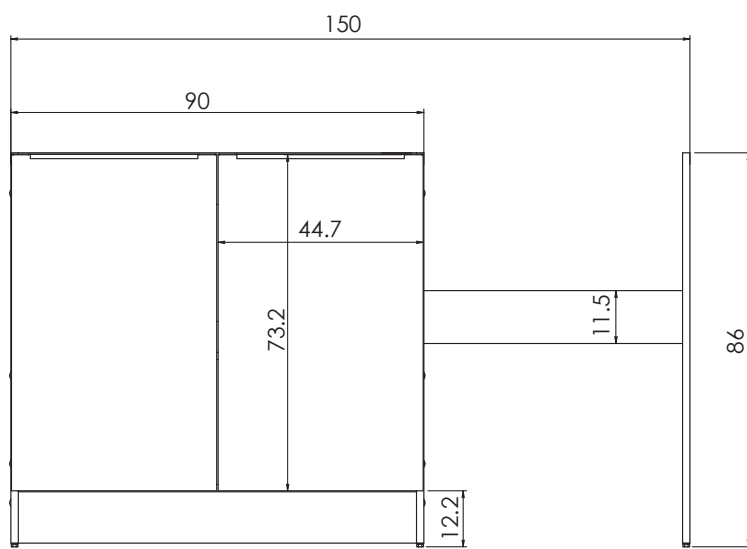
Vue face
