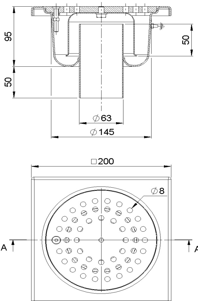
COUPE A-A
