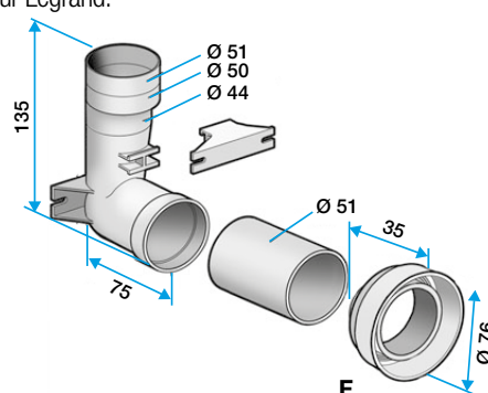
Encombrement contre-prise filaire Celiane
