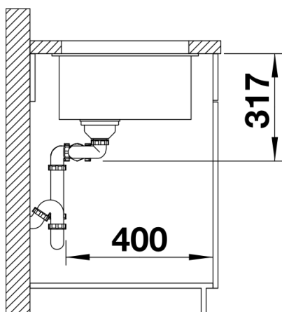
Vue latérale
