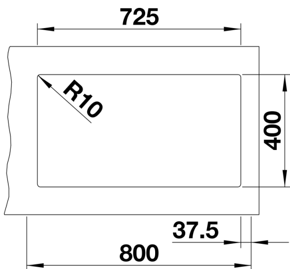
Découpe
