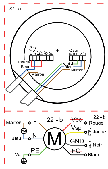
Détail câblage Ventilateur
