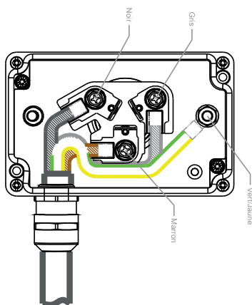
Raccordement électrique compresseur Copeland tri ZH09
