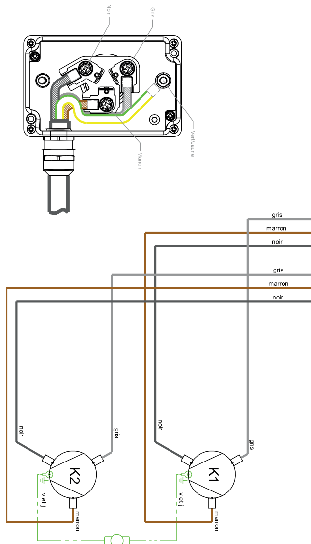
Raccordement électrique compresseur Copeland tri
