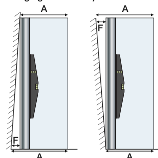
Réglage du faux-aplomb du mur
