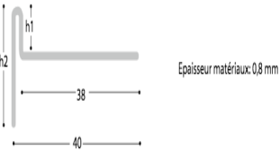
PROFILÉ I-DRAIN (Version droite); Inox, Brossé (1.4301)
