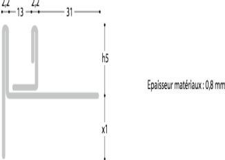
PROFILE I-DRAIN-POUR PAROI VITREE (Version droite); Inox, brossé (1.4301)
