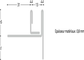
PROFILE I-DRAIN-POUR PAROI VITREE (Version gauche); Inox, brossé (1.4301)
