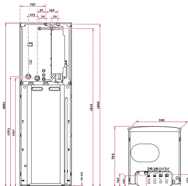
Vue arrière
