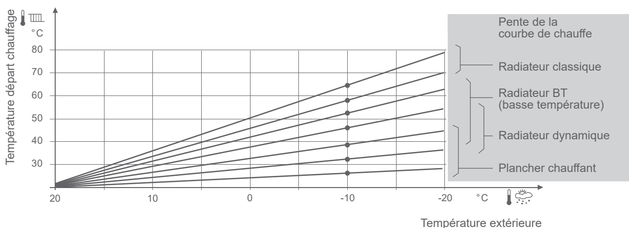
fig. 12 - Pente de la courbe de chauffe
