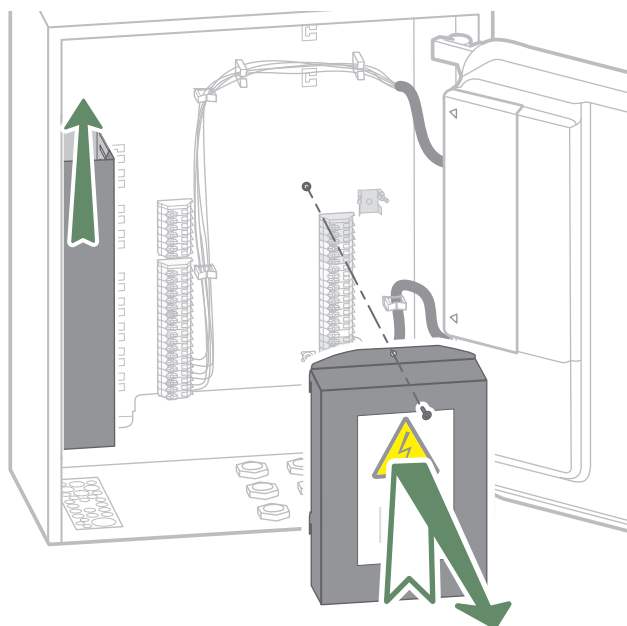
fig. 10 - Accès aux borniers
