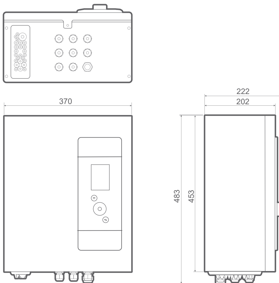
fig. 2 - Dimensions en mm
