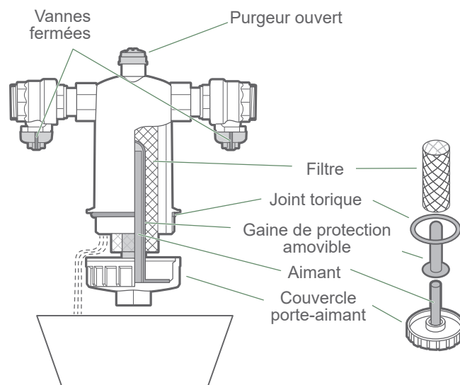
fig. 13 - Nettoyage du pot à boues
