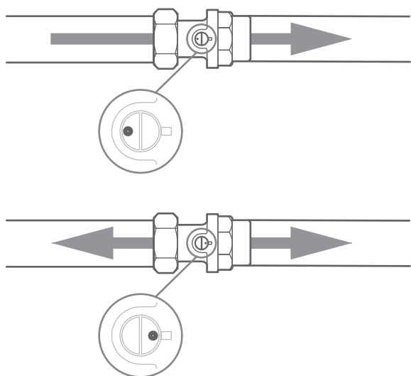
fig. 8 - Clapet antiretour
