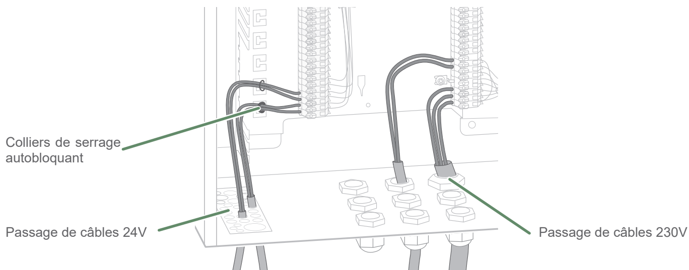
fig. 11 - Passage de câbles
