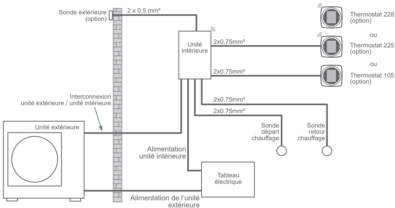
fig. 9 - Schéma d'ensemble des raccordements électriques pour une installation simple (1 circuit de chauffage)
