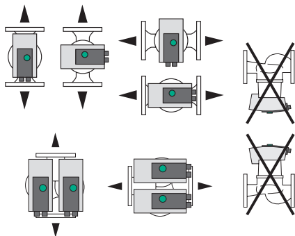
Fig. 2: Positions de montage admissibles
