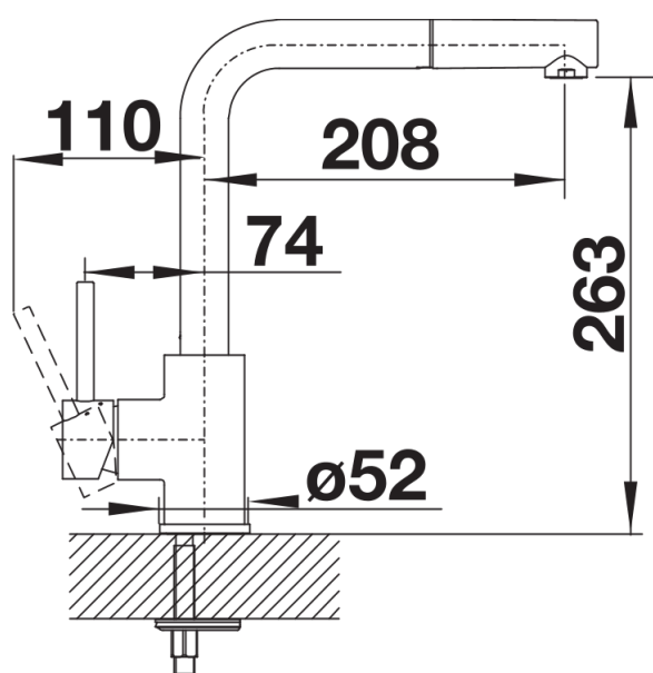
Vue latérale
