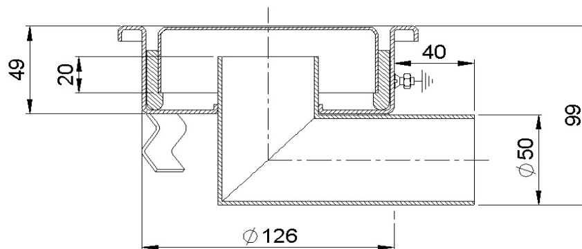
COUPE A-A
