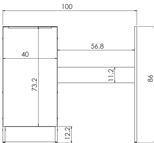
Vue face
