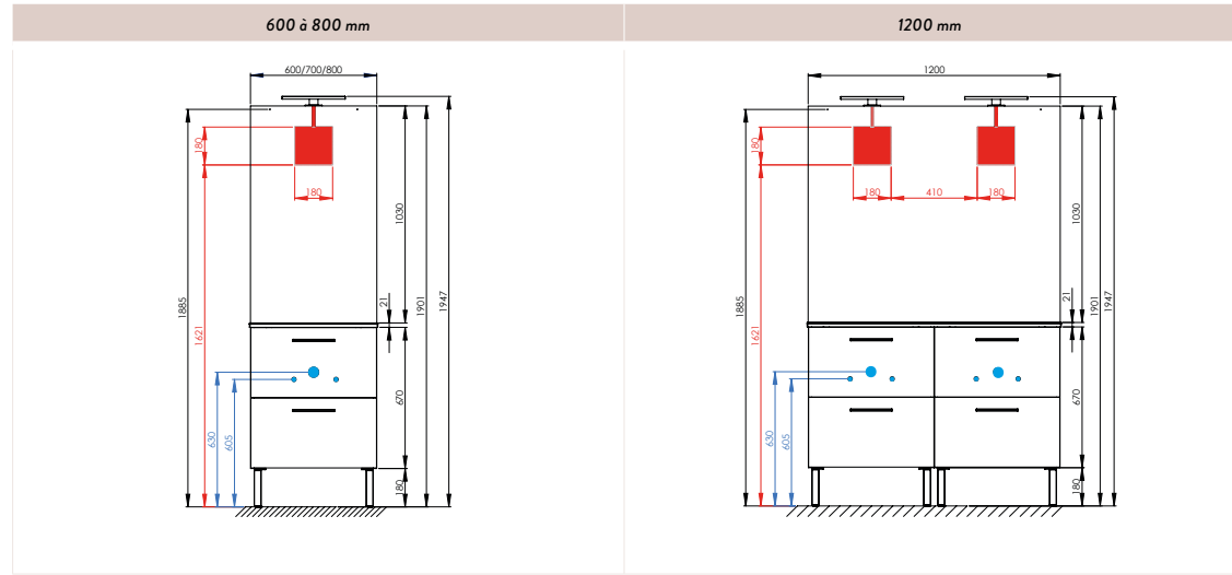
PLAN CÉRAMIQUE
