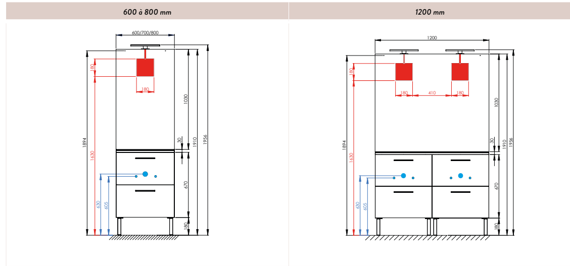
PLAN POLYBÉTON
