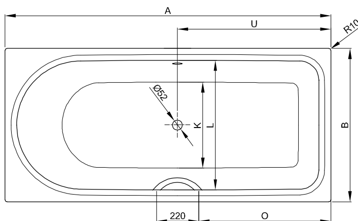
N° 1: côté pieds à droite, trop-plein derrière
