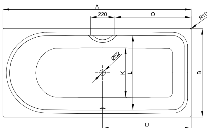
N° 2: côté pieds à droite, trop-plein devant
