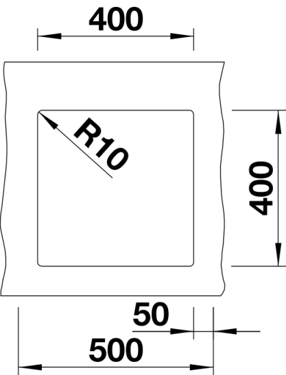
Découpe
