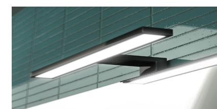
Miroir avec chants finition chromé et attaches réglables. Applique LED basse consommation, disponible en chromé et noir mat (30 W ou 50 W - 4000 K - classe énergétique A).
